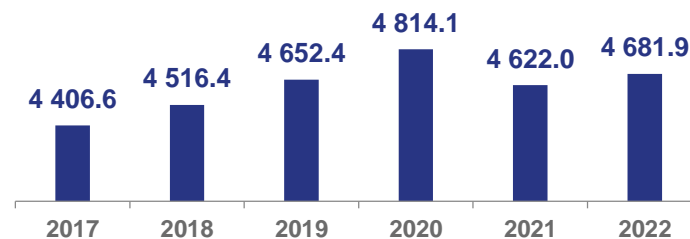
Выработано электрической энергии в 2017-2022 гг. млн кВт.ч.
